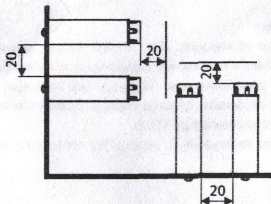
Рисунок 1 - Положения установки
