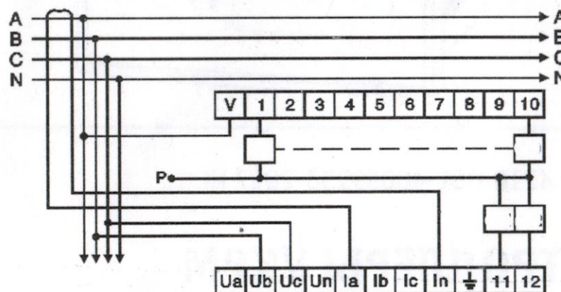
Рисунок 2. Схема подключения контроллера
