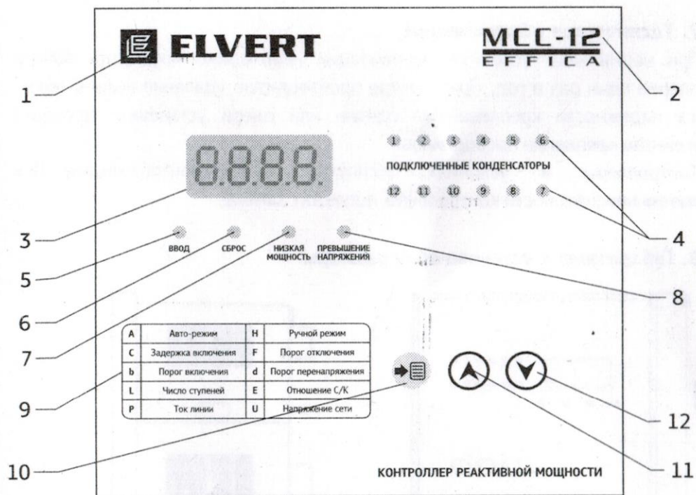
Рисунок 1. Лицевая панель контроллера
